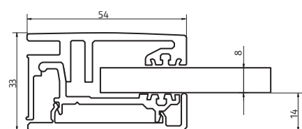
Seitenwand / Festteil
