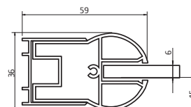
Walk In Easy Comfort Griffseite
