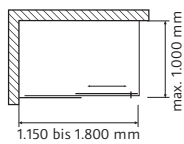
Abb.: Festelement links, Türseite rechts
