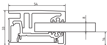
Walk In Exklusiv Wandanbindung Dreh- / Falttür
