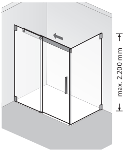
Abb.: Seitenwand rechts
