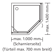
Abb.: Anschlag links
