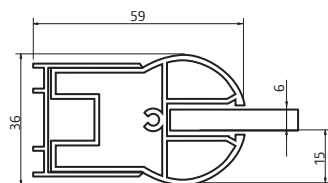
Seitenwand
